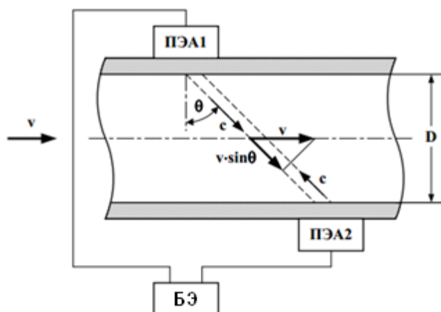
Рисунок 1 – Схема прохождения УЗС
